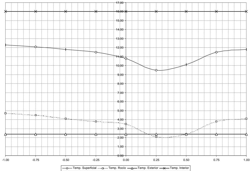
Fig. 5: Variación de temperaturas (secas y de rocío) en una sección característica de muro.
