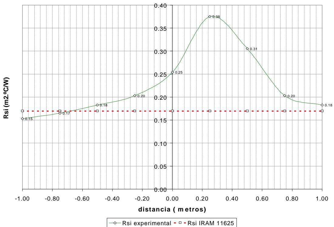
Fig. 6: Variación de la resistencia superficial exterior respecto de la establecida por la norma IRAM 11603/99 en una sección característica de muro.
