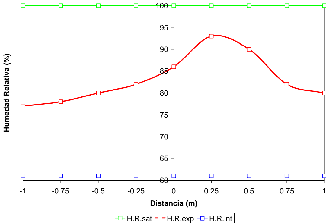
Fig. 7: Variación de la humedad relativa superficial interior en una arista de muros.
