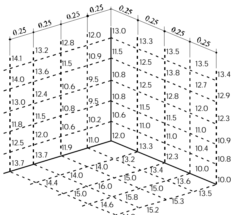
Fig. 1: Esquema de relevamiento de datos en grilla para un encuentro característico de pared / pared / piso.
