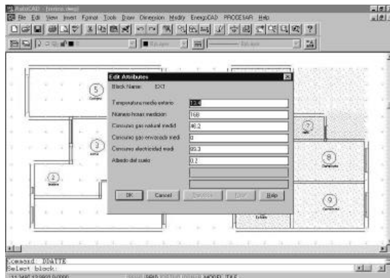
Fig. 3 Ejemplo de edición de características de un sistema constructivo
