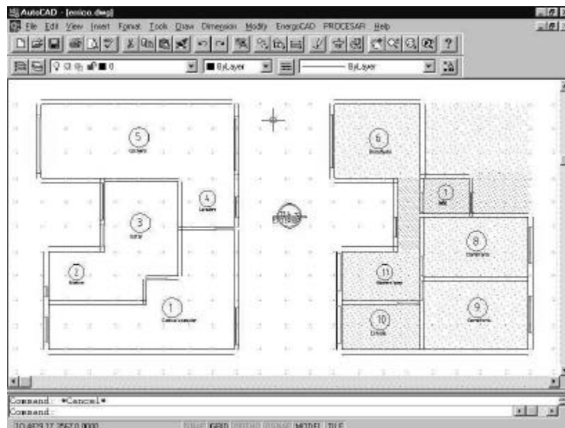
Fig. 1 Unidad de pre procesamiento gráfico del sistema AuditCAD
