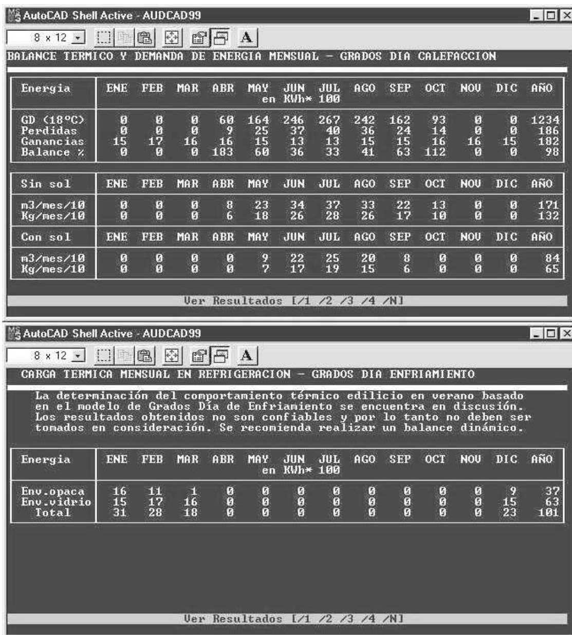
Fig. 8 Ejemplo: resultados detallados mensuales de un edificio auditado.
